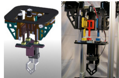
(στ) Εικονικό πρωτότυπο ρομποτικού βραχίονα και το τελικό φυσικό πρωτότυπο.
