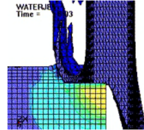
(γ) Ανάλυση και βελτιστοποίηση υδροκοπής με χρήση συστήματος FEM (Πολυτεχνείο Κρήτης, 2011).
