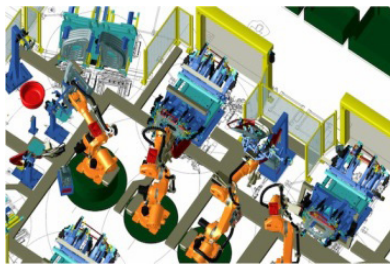
(ζ) Εικονική παραγωγή με το λογισμικό ROBOCAD.
