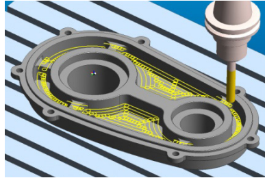
(β) Επιθυμητή σειρά των κατεργασιών και πορεία του κοπτικού εργαλείου για σύστημα CAM.
